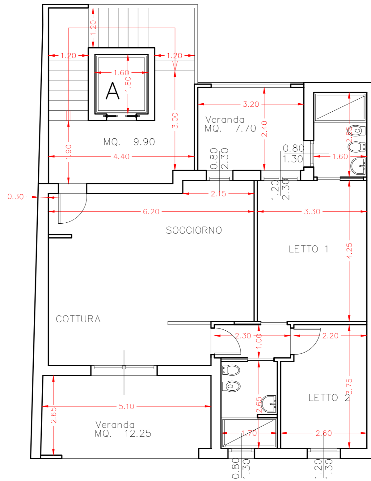
PIANTA P. 1° TRIVANO OPEN SPACE
