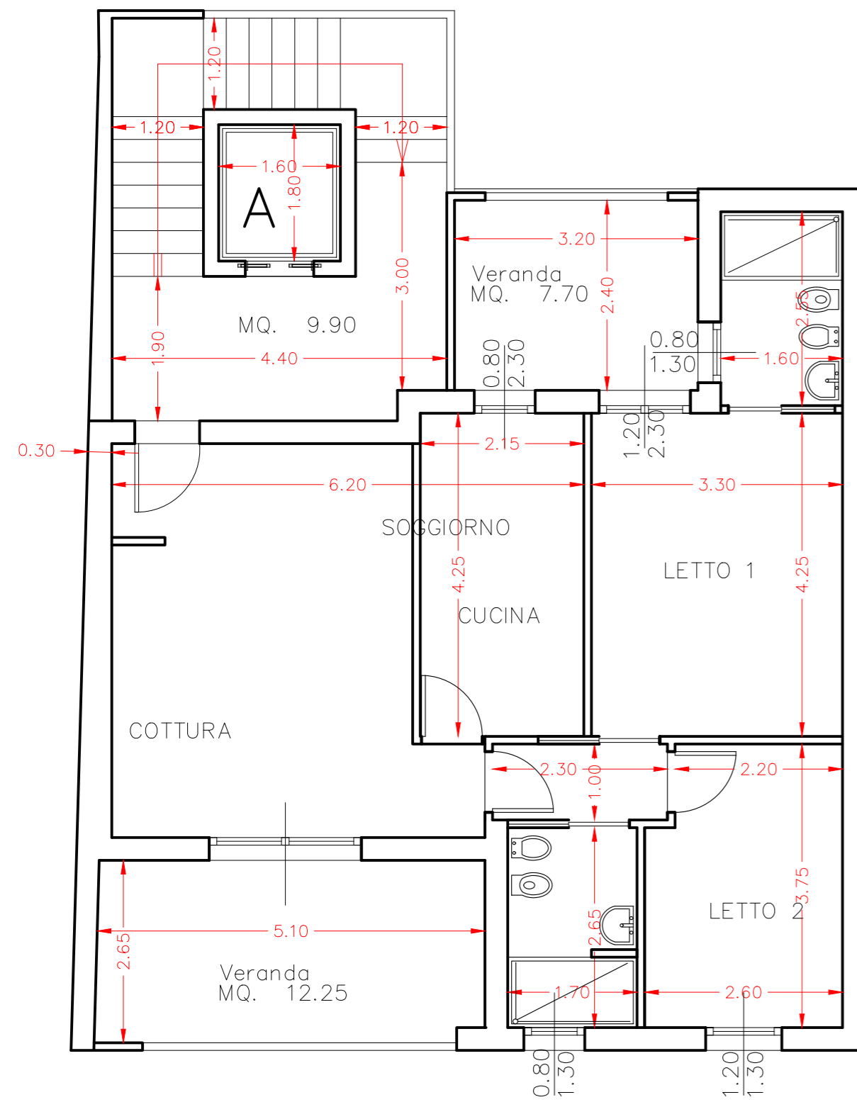
PIANTA P. 1° TRIVANO CUCINA ABITABILE
