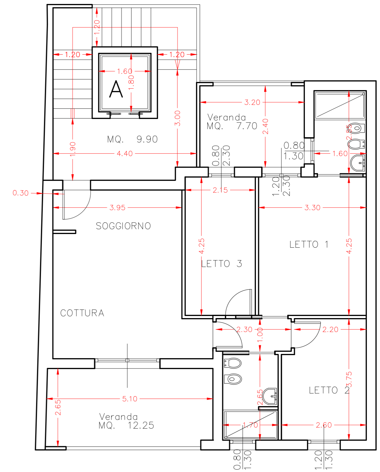
PIANTA P. 1° QUADRIVANO ANGOLO COTTURA
